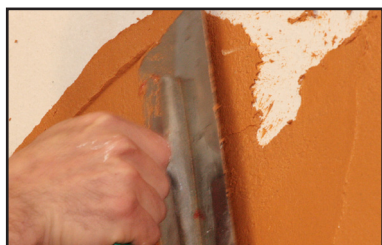
Étape 3 - application de l'enduit en 3/4 mm à l'aide d'une spatule inox.
